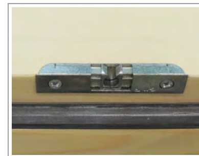
SCHNÄPPER Halter optional mit ETÖ Oben montiert!
