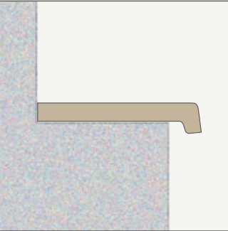
Klassische Variante mit vorstehender Fensterbanknase
