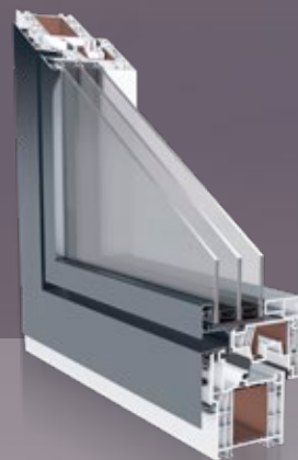
MyUnity PURO Flügel flächenbündig, Glaseinsatz leicht rückspringend
