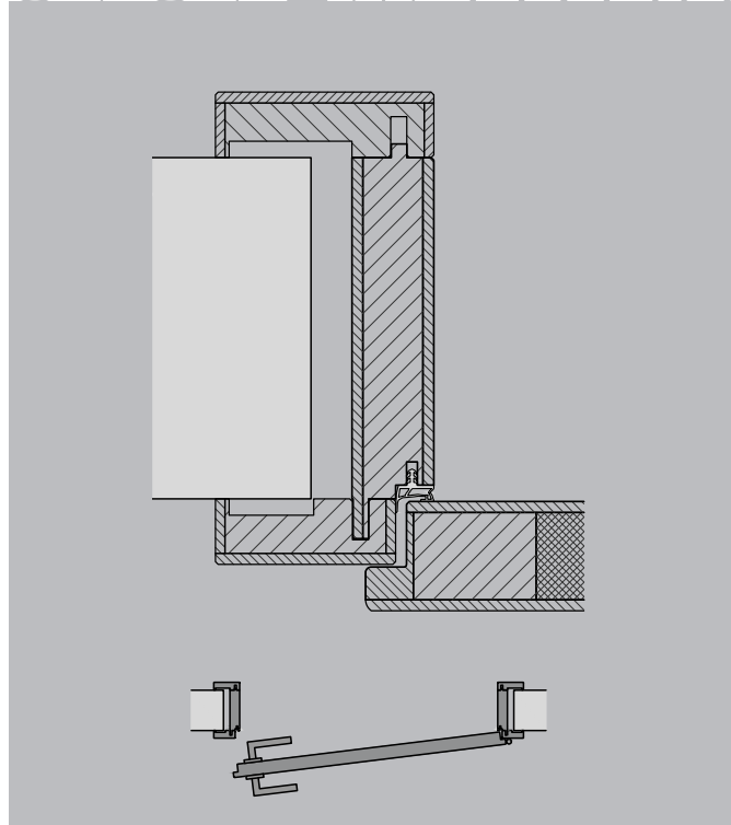
F4F1 Türblatt überfält Abbildung Natura Massiv
