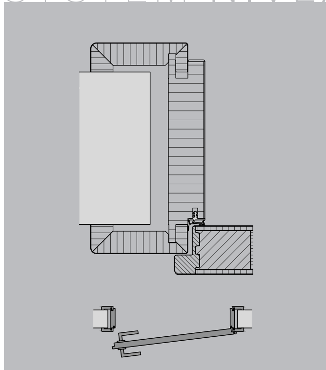
FF1 Türblatt überfäلت Abbildung furniert
