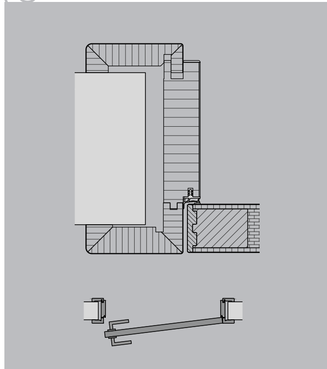
FB1E bündig einschlagend Abbildung furniert
