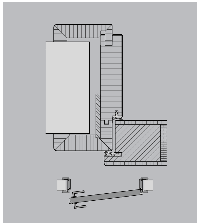
FF2T Abschlusstürblatt, Doppeldichtung Türblatt überfäلت Abbildung furniert
