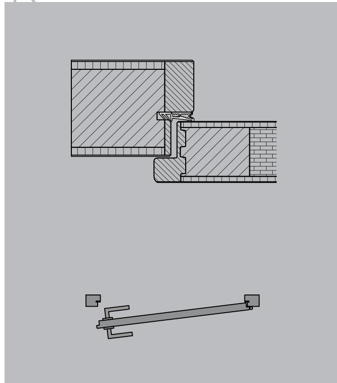
PF1 Türblatt überfäلت Abbildung furniert
