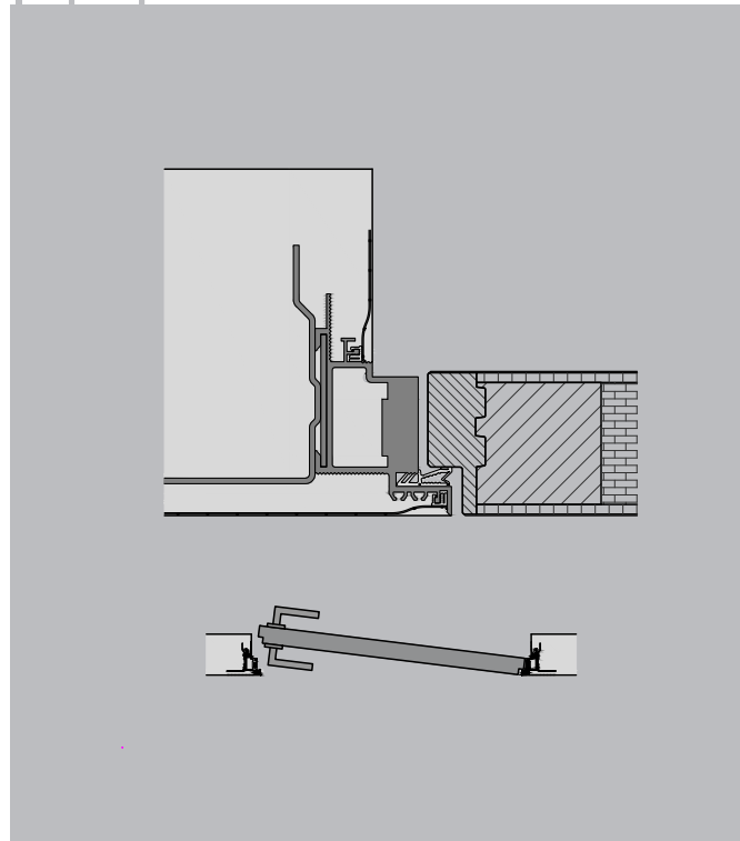
UR6 Öffnung Laibungsseite Abbildung furniert
