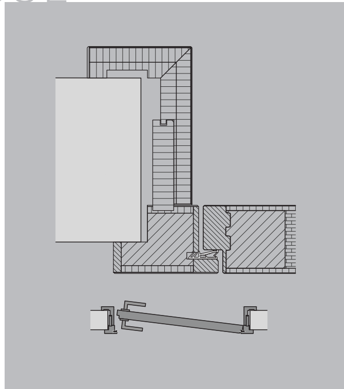
F3R1 Return – in Laibung öffnend Abbildung furniert
