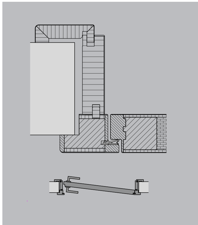
FR1 Return – in Laibung öffnend Abbildung furniert
