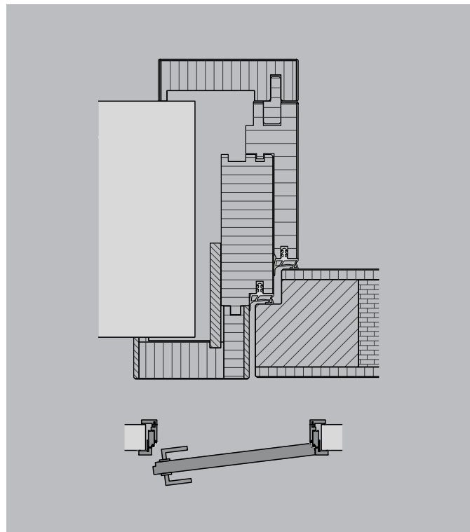
F4B4T Abschlussstürblatt, Doppeldichtung bündig einschlagend Abbildung furniert
