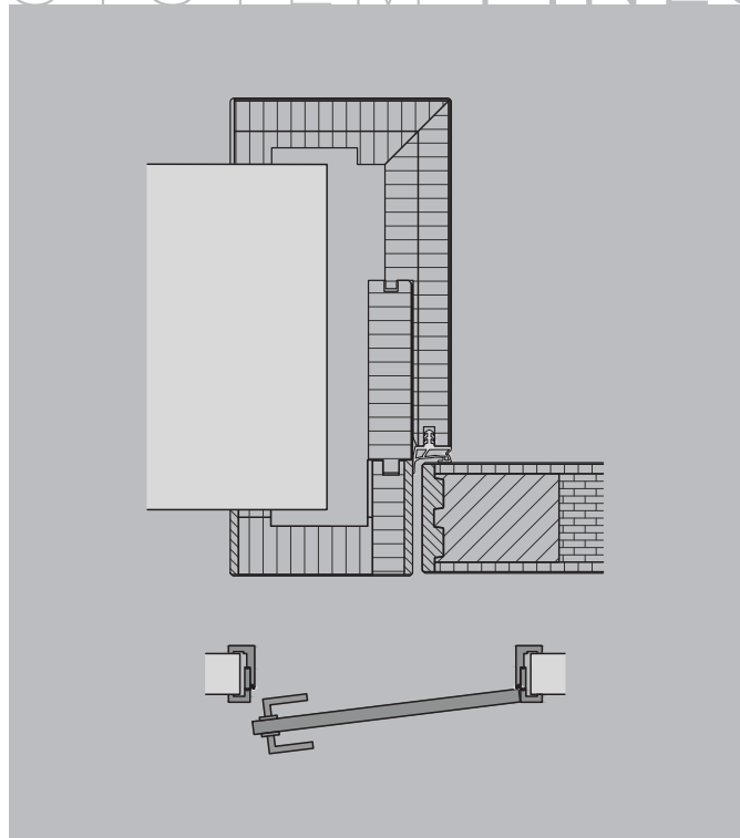
F3B1E bündig einschlagend Abbildung furniert
