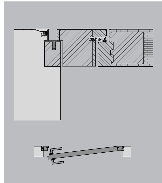
PB2E beidseitig flächenbündig Abbildung furniert
