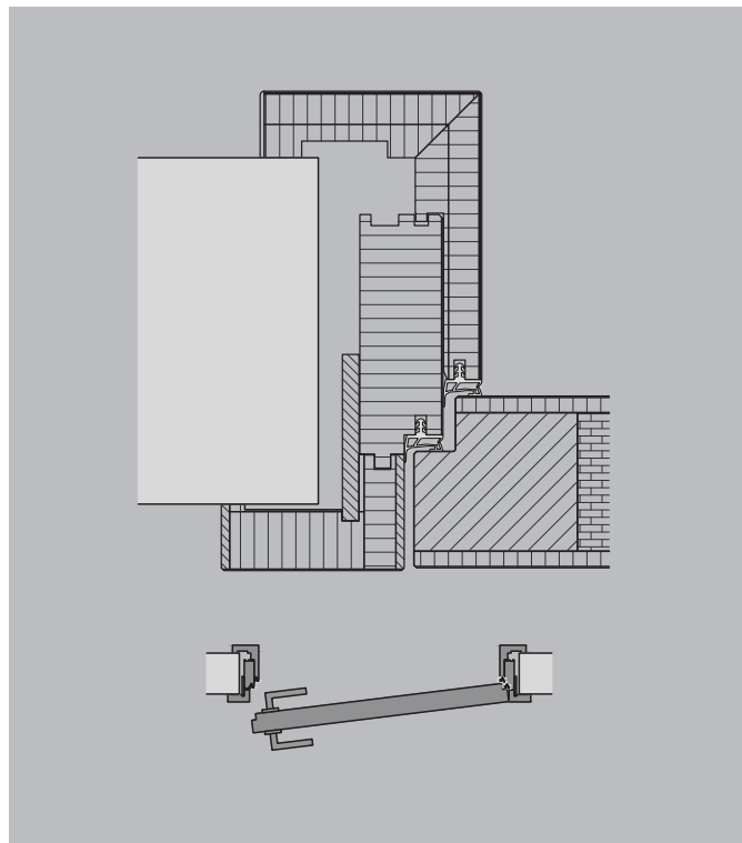
F3B4T Abschlussstürblatt, Doppeldichtung bündig einschlagend Abbildung furniert
