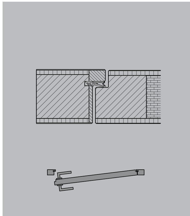
PB2T Abschlusstürblatt beidseitig flächenbündig Abbildung furniert
