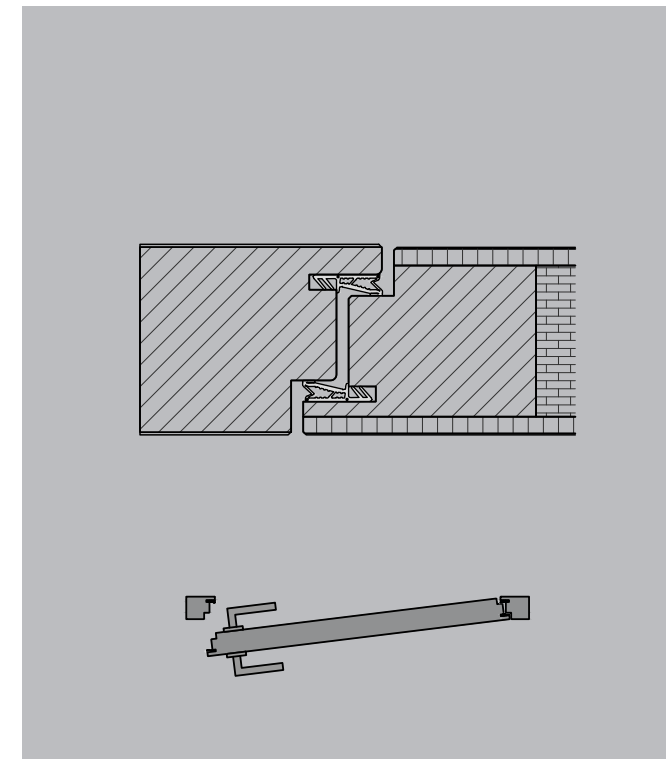
PB3T Abschlusstürblatt, Doppeldichtung beidseitig flächenbündig Abbildung furniert
