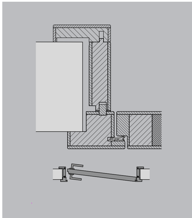
F4R1 Return – in Laibung öffnend Abbildung Natura Massiv
