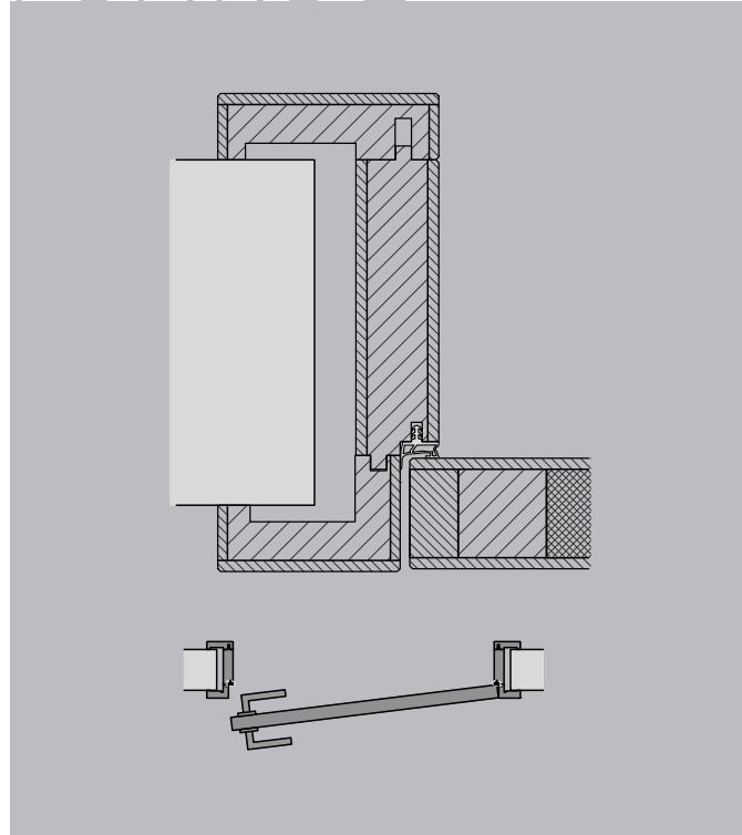
F4B1E bündig einschlagend Abbildung Natura Massiv
