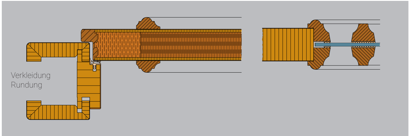
| PROFIL F1
