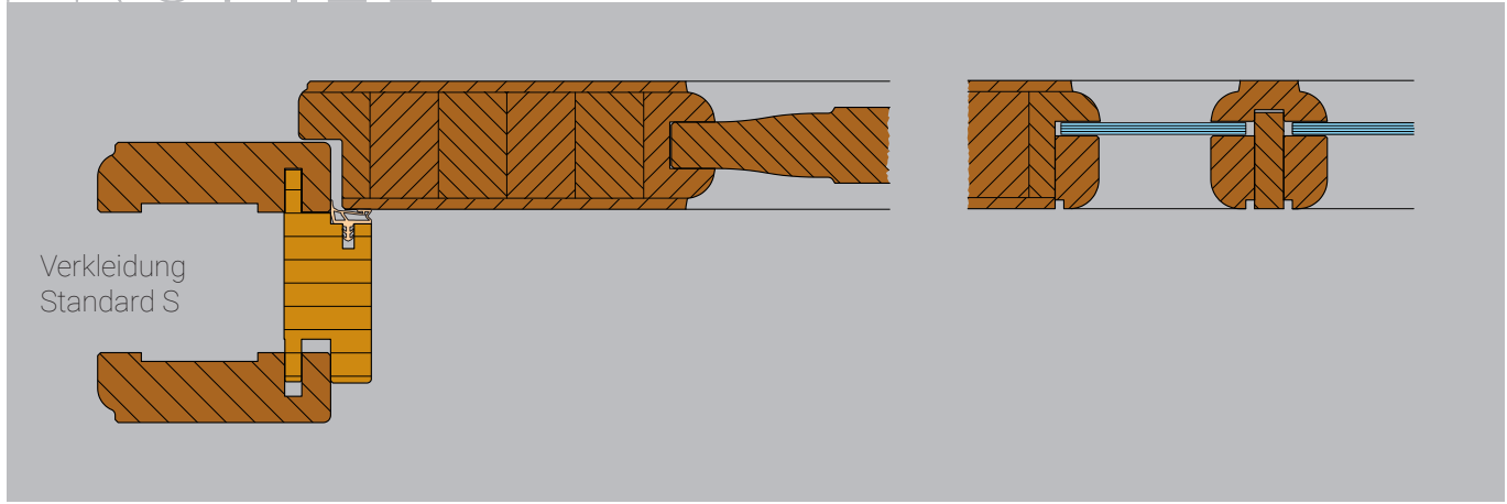
| PROFIL K1
