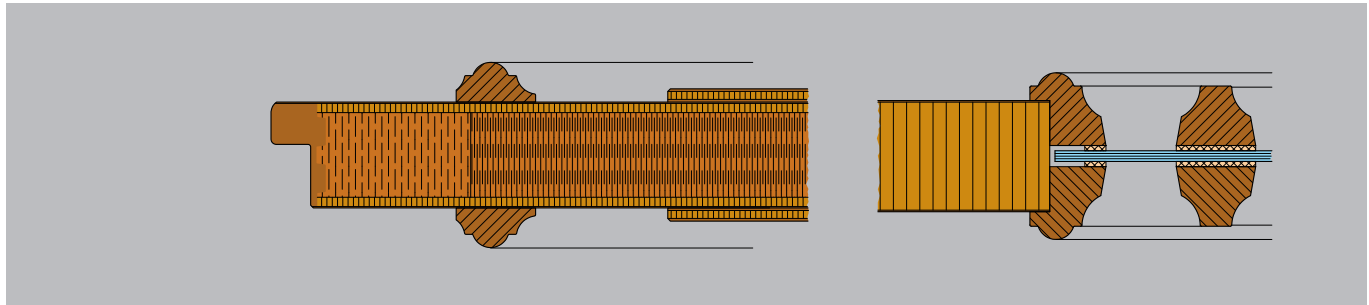
| PROFIL F6
